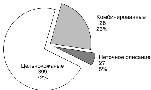
Рис. 2. Переплеты книг
